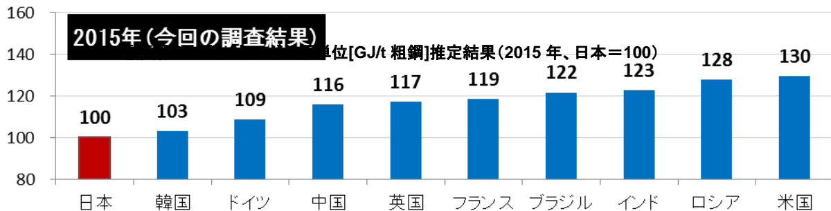
電炉鋼の一次エネルギー原単位[GJ/t 粗鋼]推定結果(2015 年、日本=100)
