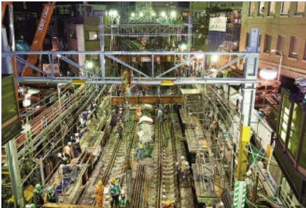
2013年3月 東急東横線渋谷～代官山間地下工事
