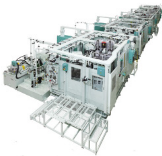
乗用四輪自動車ナックル加工ライン 異形なショートナックルを高効率生産
