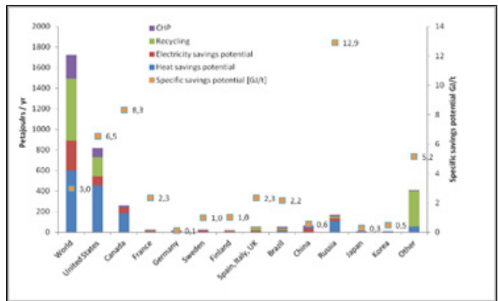
図 8 利用可能な最善技術(BAT)を利用した場合の省エネ可能ポテンシャルの国際比較
