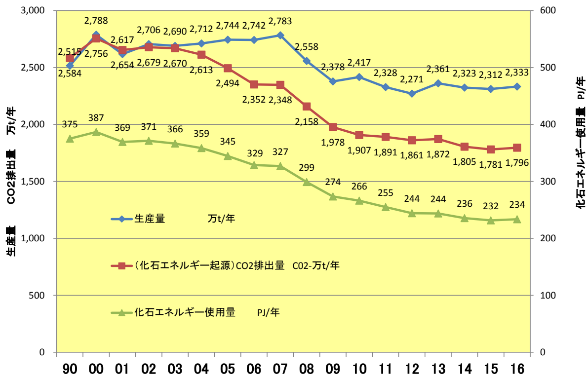
図1 生産量とCO 2 排出量および化石エネルギー使用量の推移
