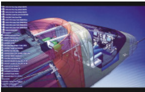
当社ソフトウェアで設計したソーラー・インパルスのコックピット。最長5日間の単独飛行に耐える操縦空間と機体の軽量化を両立している 提供：Dassault Systèmes
